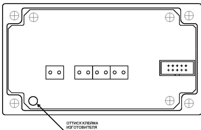
Рисунок 4.3 – Места пломбирования
