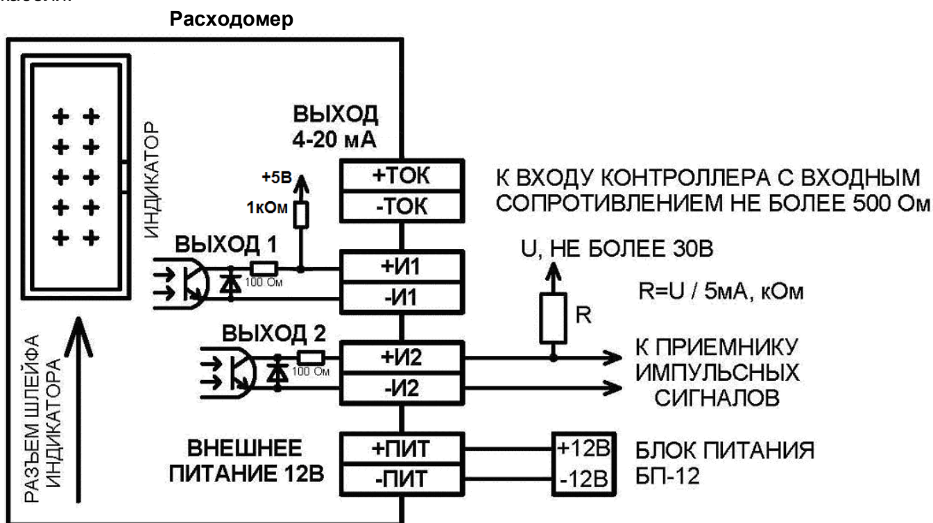
Рисунок 4.2 – Подключение к ЭМР
