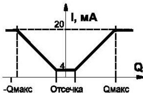
Рисунок 4.5 - Выходная характеристика токового выхода
